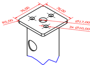
A ( 1 : 2 )
